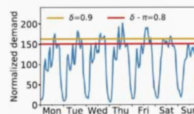
Рис. 2. Пики нагрузки группы приложений со схожими требованиями к сети на периферийных узлах сети доступа Источник: Resource Sharing Efficiency in Network Slicing
