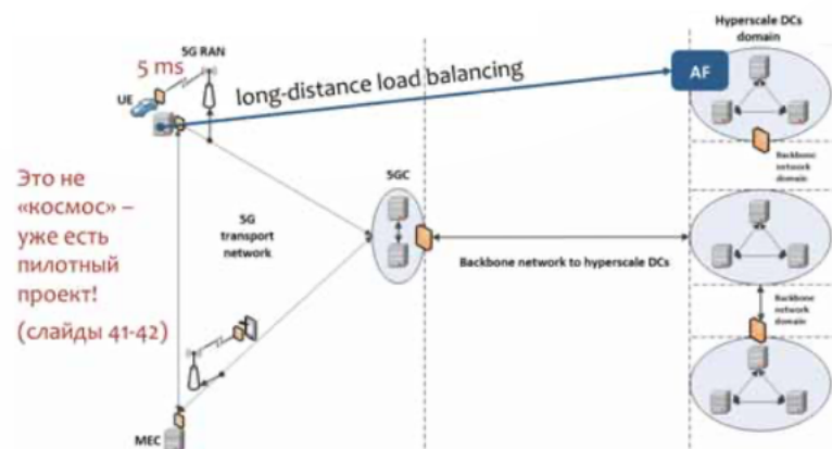
Рис. 3. Балансировка нагрузки в кросс-доменном сетевом слое
